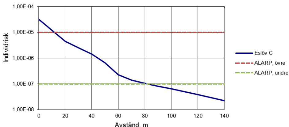
Figur 6 - Individrisk som funktion av avståndet från närmaste räl. Individrisken gäller utifrån både Marieholmsbanan och Södra stambanan. Utredningsområdet ligger som närmast 120 m avstånd från närmsta räl.
