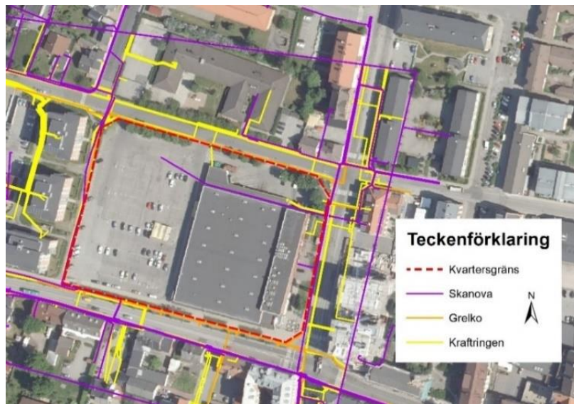
Övriga ledningar som kan komma att behöva tas hänsyn till vid exploatering av planområde.
