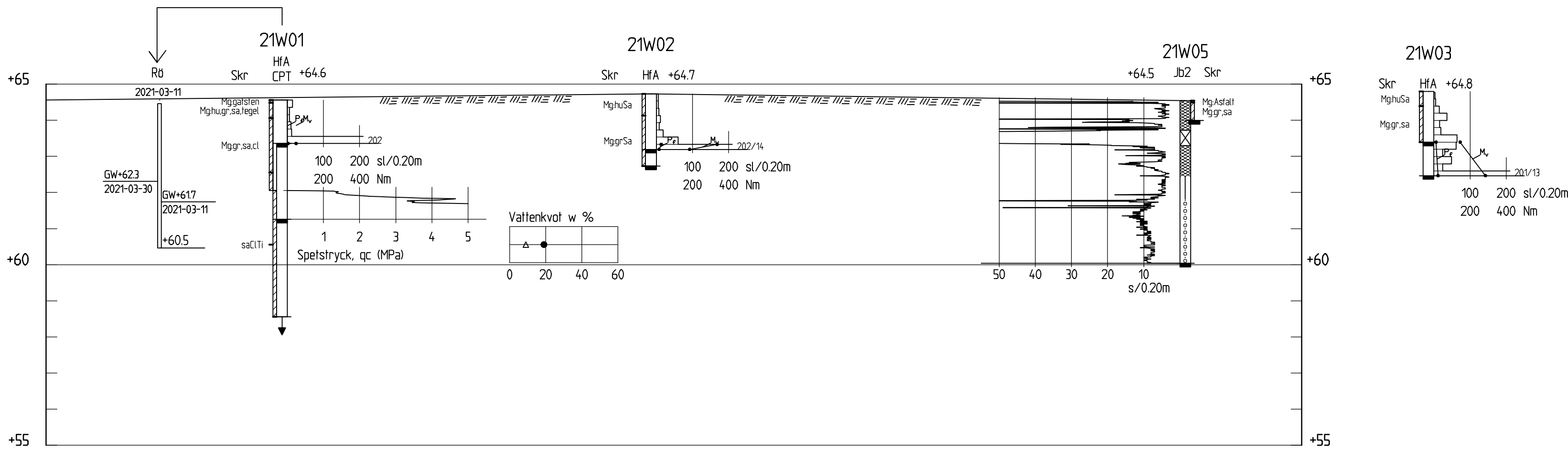
SEKTION A-A 1: 100
