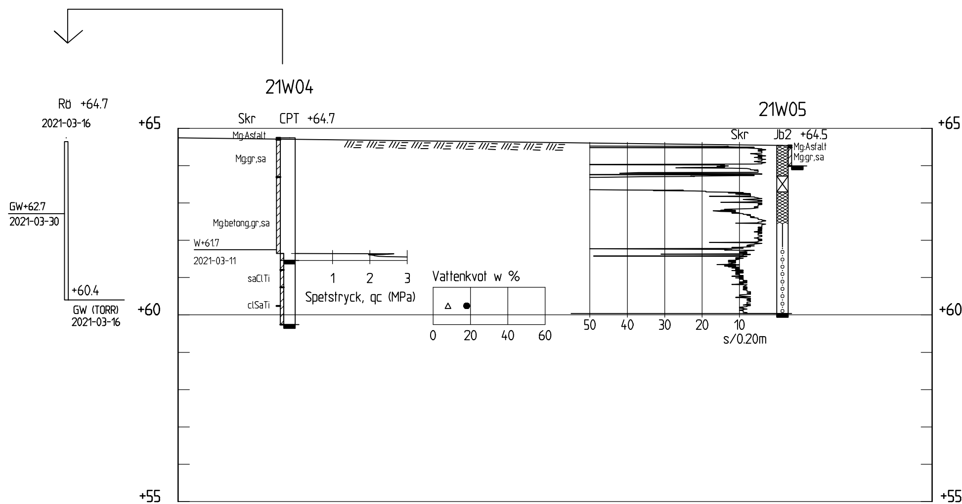
SEKTION B-B 1: 100
